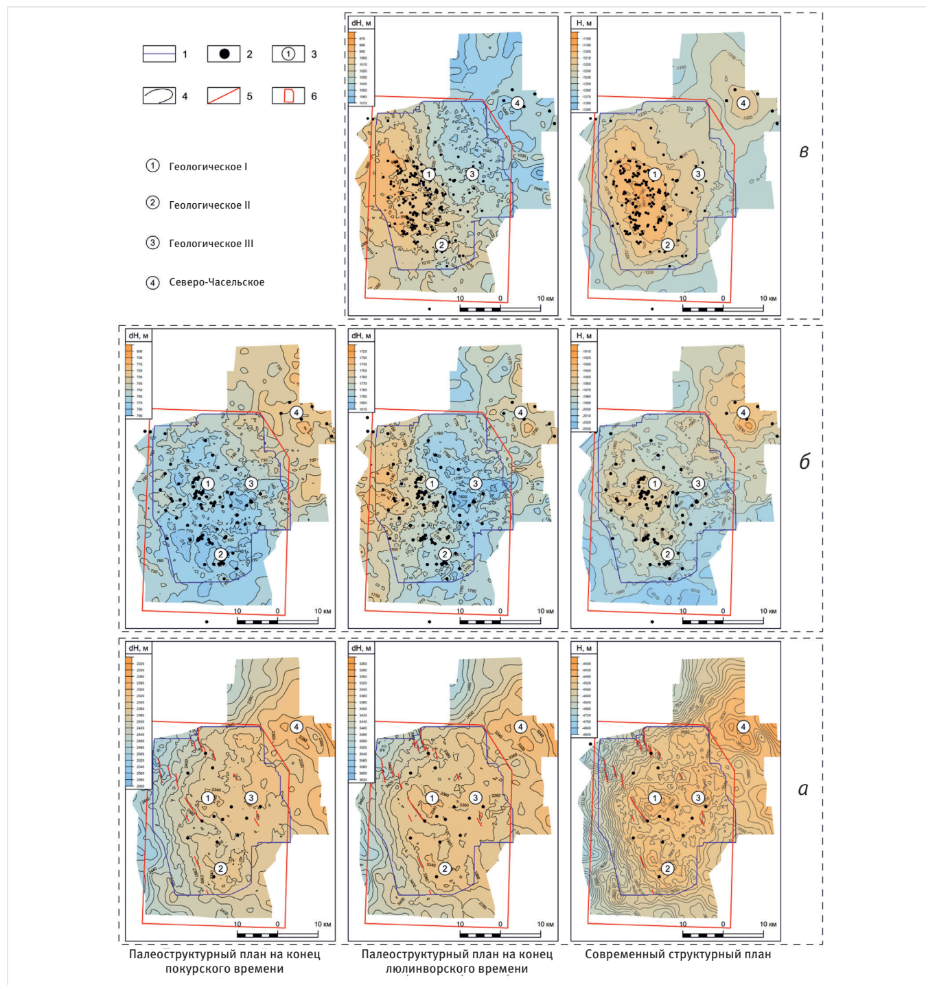
Рис. 1. История формирования структурных планов а — ОГ Т, б — М', в — Г на конец покурского времени, люлинворского времени и их современный облик.
