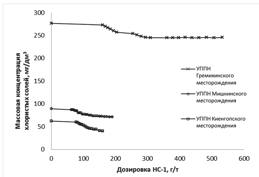
Рис. 3. Зависимость содержания хлористых солей от дозировки НС-1 для товарных нефтей УППН Киенгопского, УППН Мишкинского и УППН Гремихинского месторождений при определенных температурно-временных характеристиках объектов Fig. 3. The dependence of the content of chloride salts on the dosage of NS-1 for commercial oils UPPN Kiengopskoye, UPPN Mishkinskoye and UPPN Gremikhinskoye fields at certain temperature and time characteristics of objects
