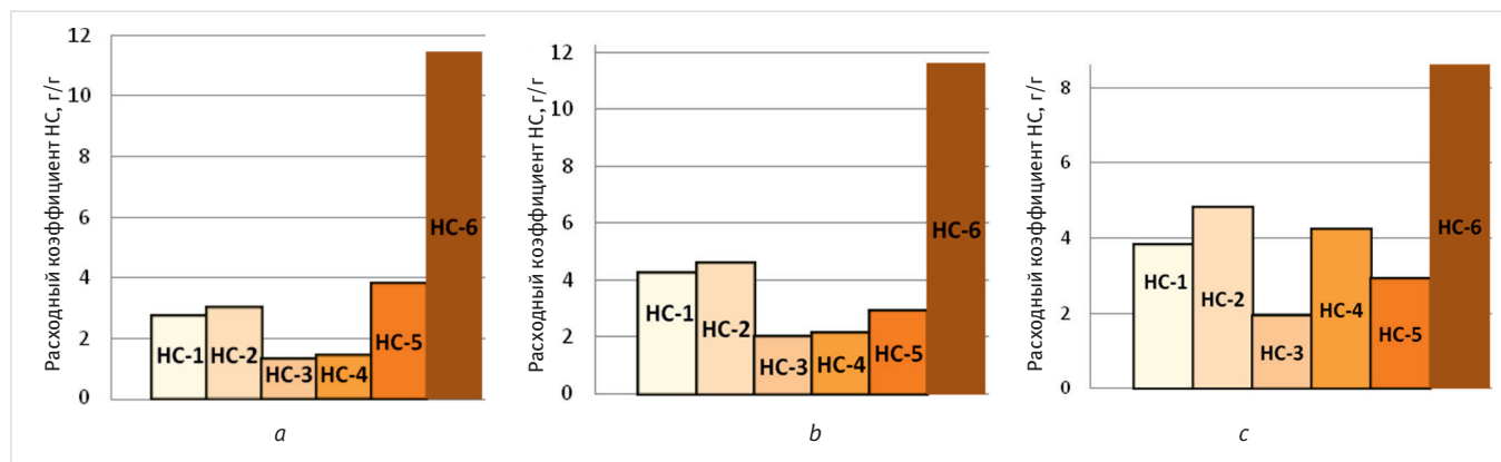
Рис. 2. Результаты определения расходного коэффициента разных марок нейтрализаторов сероводорода для нефтей с УППН Киенгопского месторождения — а, УППН Мишкинского месторождения — б, УППН Гремихинского месторождения — с Fig. 2. The results of determining the consumption coefficient of different grades of hydrogen sulphide neutralizers for oils from the UPPN Kiengopskoye field — а, UPPN Mishkinskoye field — б, USPН Gremikhinskoye field — с
