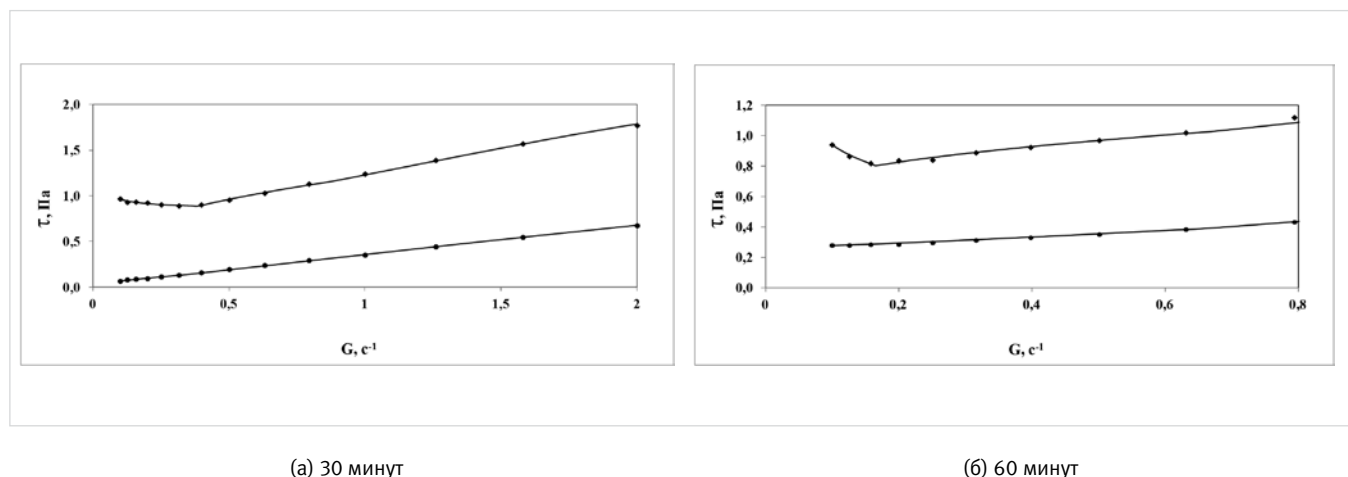
Рис. 2 — Зависимости \tau(G) для случая, когда после роста G от 0,1 \text{ с}^{-1} до G=100 \text{ с}^{-1} , воздействие скоростью сдвига было остановлено на 30 (а) и 60 (б) мин., а затем была снята зависимость \tau(G) при снижении G от 100 \text{ с}^{-1} до 0,1 \text{ с}^{-1} . Точки — экспериментальные данные, сплошные линии расчет по формуле (4) Fig. 2 — Dependence \tau(G) for the case when, after increasing G from 0.1 \text{ с}^{-1} to G=100 \text{ с}^{-1} , the exposure of the shear rate was stopped for 30 (a) and 60 (b) minutes, and then the dependence \tau(G) was registered when G decreased from 100 \text{ с}^{-1} to 0.1 \text{ с}^{-1} . Points-experimental data, solid lines calculation using the formula (4)
