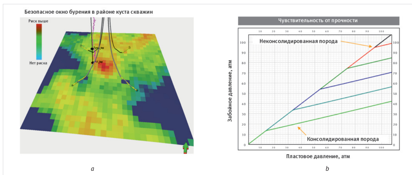
Рис. 2. Безопасное окно бурения по площади одной из кустовых площадок — а и зависимость безопасной депрессии от прочности при эксплуатации скважины — б Fig. 2. Safe drilling window over the area of one of the well pads — а and dependence of safe drawdown on strength during well operation — б
