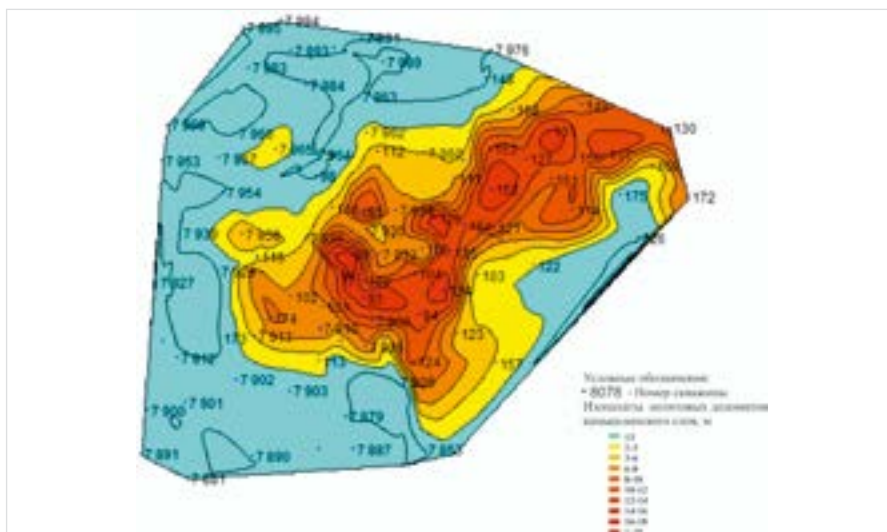
Рис. 2 — Карта изопакит оолитовых доломитов камышлинского слоя. Масштаб 1:50000. Fig. 2 — Thickness map of oolite dolomite Kamyshla beds. Plotscale 1:50000.
