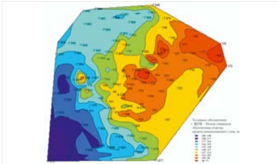
Рис. 1 — Структурная карта по кровле камышлинского слоя. Масштаб 1:50000. Fig. 1 — Structural map of the roof Kamyshla beds. Plot scale 1:50000.
