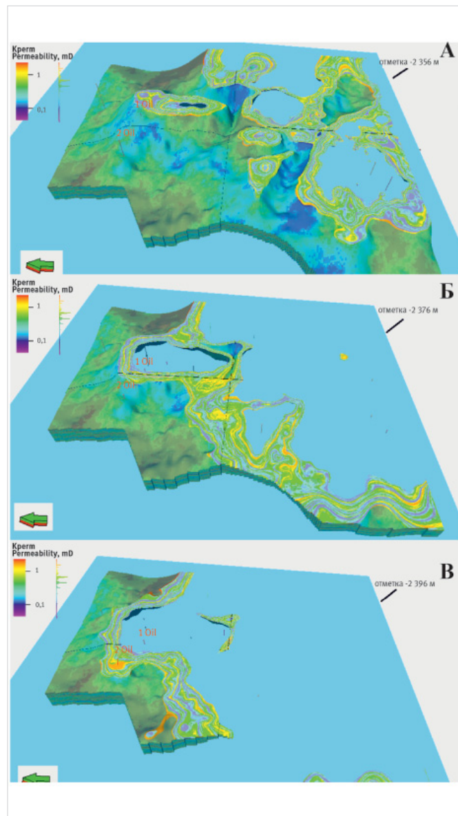
Рис. 7. 3D-модели пласта AC_{12} для пропластков AC_{12}^1 , AC_{12}^2 , AC_{12}^3 (параметр «проницаемость») 1 — плоскость среза параметра «проницаемость» на каждые 20 м от кровли пласта (2 296 м) (А, Б, В). Скважины 1 Oil и 2 Oil, предлагаемые к бурению Fig. 7. 3D model of the AC_{12} formation for the AC_{12}^1 , AC_{12}^2 , AC_{12}^3 interlayers ("permeability" parameter) 1 — plane of cut of the parameter "permeability" for every 20 meters from the top of the reservoir (2 296 m) (A, B, B). Wells 1 Oil and 2 Oil proposed for drilling
