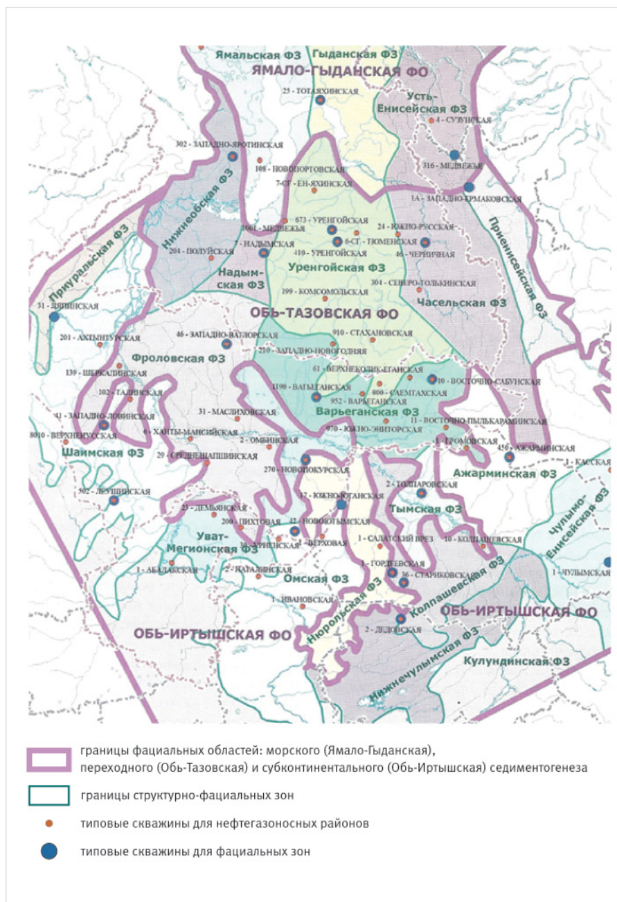
Рис. 1. Схема фациальных районов отложений Западной Сибири [1] Fig. 1. Scheme of facies regions of deposits of Western Siberia [1]
