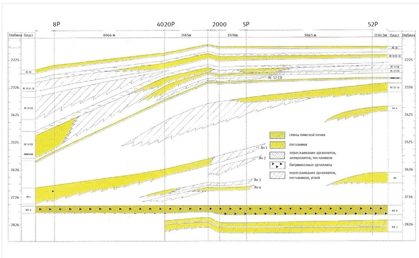
Рис. 2. Палеогеологический разрез верхнеюрских-нижнемеловых отложений на Ай-Пимском месторождении, по данным [7] Fig. 2. Paleogeological section of the Upper Jurassic-Lower Cretaceous deposits at the Ai-Pimskoye field according to the data [7]
