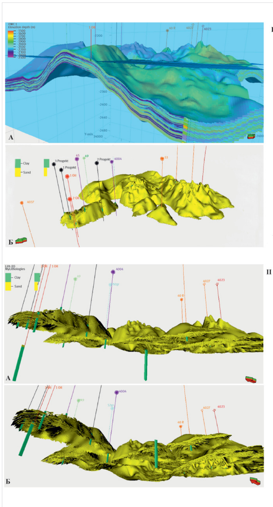
Рис. 4. Граница ВНК для продуктивной части пласта AC_{12}^1 I. А — граница ВНК в пределах Ай-Пимского и Западно-Чигоринского месторождений; Б — Куб NTG. «Отсечение» продуктивной части AC_{12}^1 ВНК, наличие песчаной фракции (количественное) II. А — распространение песчаных фракций в меридиональном направлении; Б — та же модель, повернутая «выше» к альтитуде устья, для наглядности изображения сложности строения пласта Fig. 4. OWC boundary for the productive part of the AC_{12}^1 formation I. A — OWC border within the Ai-Pimskoye and Zapadno-Chigorinskoye fields; Б — NTG Cube. “Cutting off” of the productive part of the AC_{12}^1 OWC, the presence of the sand fraction (quantitative) II. A — distribution of sand fractions in the meridional direction; Б — the same model, turned “higher” to the wellhead altitude, for clarity of depicting the complexity of the reservoir structure
