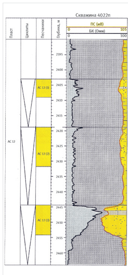
Рис. 3. Строение пласта AC 12 в скважине 4022 на Ай-Пимском месторождении [7] Fig. 3. Structure of the AC 12 formation in well 4022 at the Ai-Pimskoye field [7]
