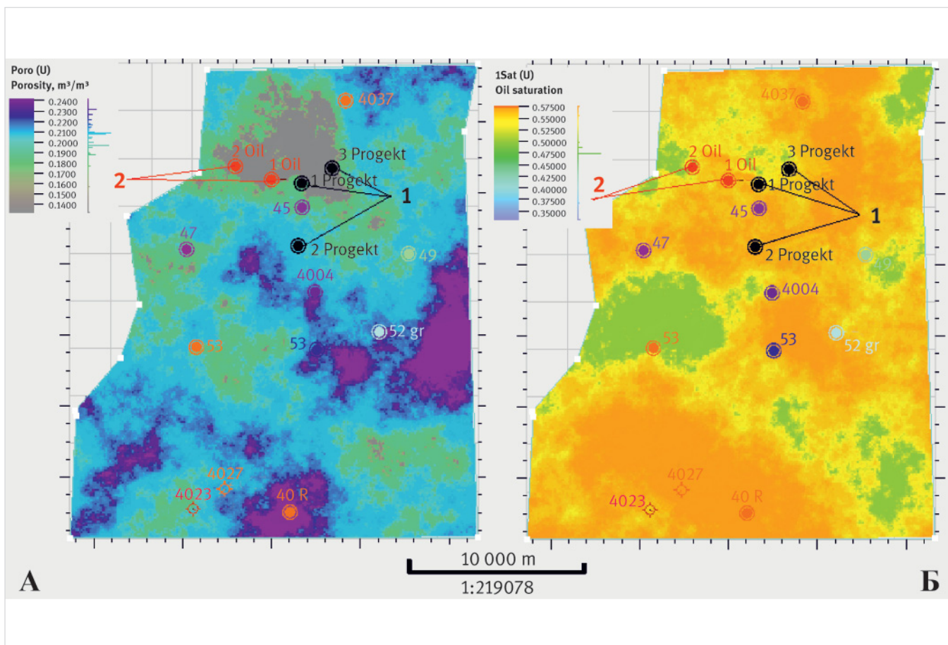
Рис. 5. 2D-модели пласта AC_{12} для пропластка AC_3^3 А — параметр «пористость»; Б — параметр «проницаемость»; 1 — скважины, пробуренные в 2019 г.; 2 — скважины, предлагаемые к бурению Fig. 5. 2D model of the AC_{12} reservoir for the AC_3^3 interlayer А — parameter «porosity»; Б — parameter «permeability»; 1 — wells drilled in 2019; 2 — wells proposed for drilling
