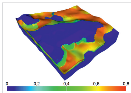
Рис. 1. Куб нефтенасыщенности по кровле коллектора Fig. 1. Oil saturation cube on the top of the reservoir
