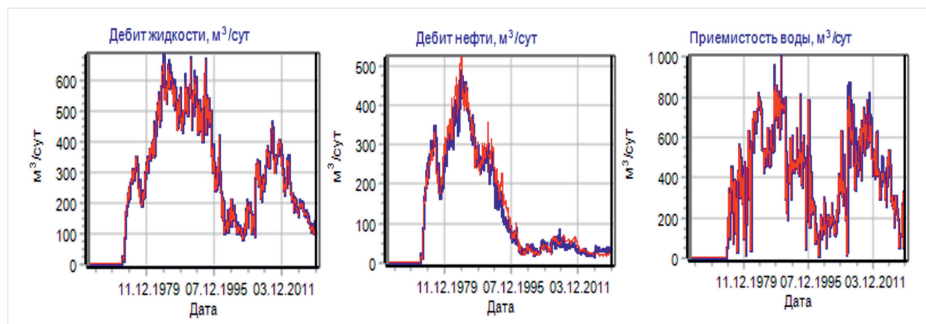
Рис. 2. Результаты адаптации ГДМ (синий график — фактические параметры; красный график — расчетные параметры) Fig. 2. HDM adaptation results (blue graph — actual parameters; red graph — calculated parameters)
