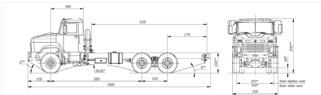
Базовый вариант с кабиной КрАЗ (с учетом переноса топливных баков и элементов выхлопной системы)
